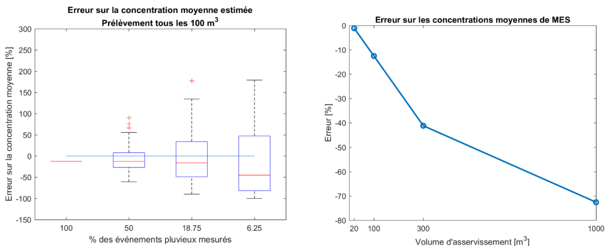
Figure 1 : À gauche, Estimation de l'incertitude en fonction du pourcentage de pluie échantillonnées. À droite, Erreurs de représentativité temporelle de la méthode OFROU en fonction du volume d'asservissement, avec toutes les pluies échantillonnées.
